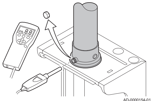
ábra39 Füstgázmérő csomak
