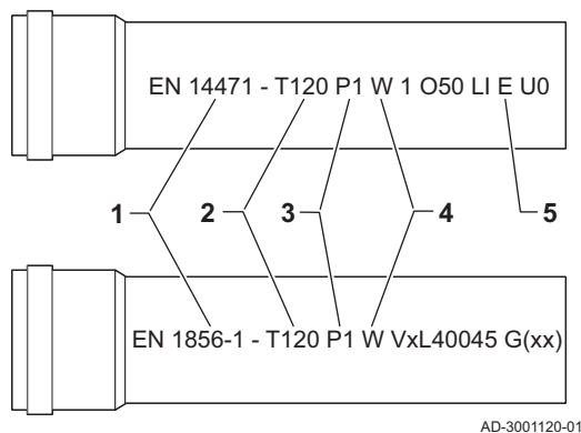
ábra4 Minta karakterlánc
