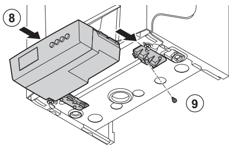
ábra22 A csatlakozódoboz felszerelése
