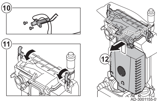
ábra67 Szétszerelés
