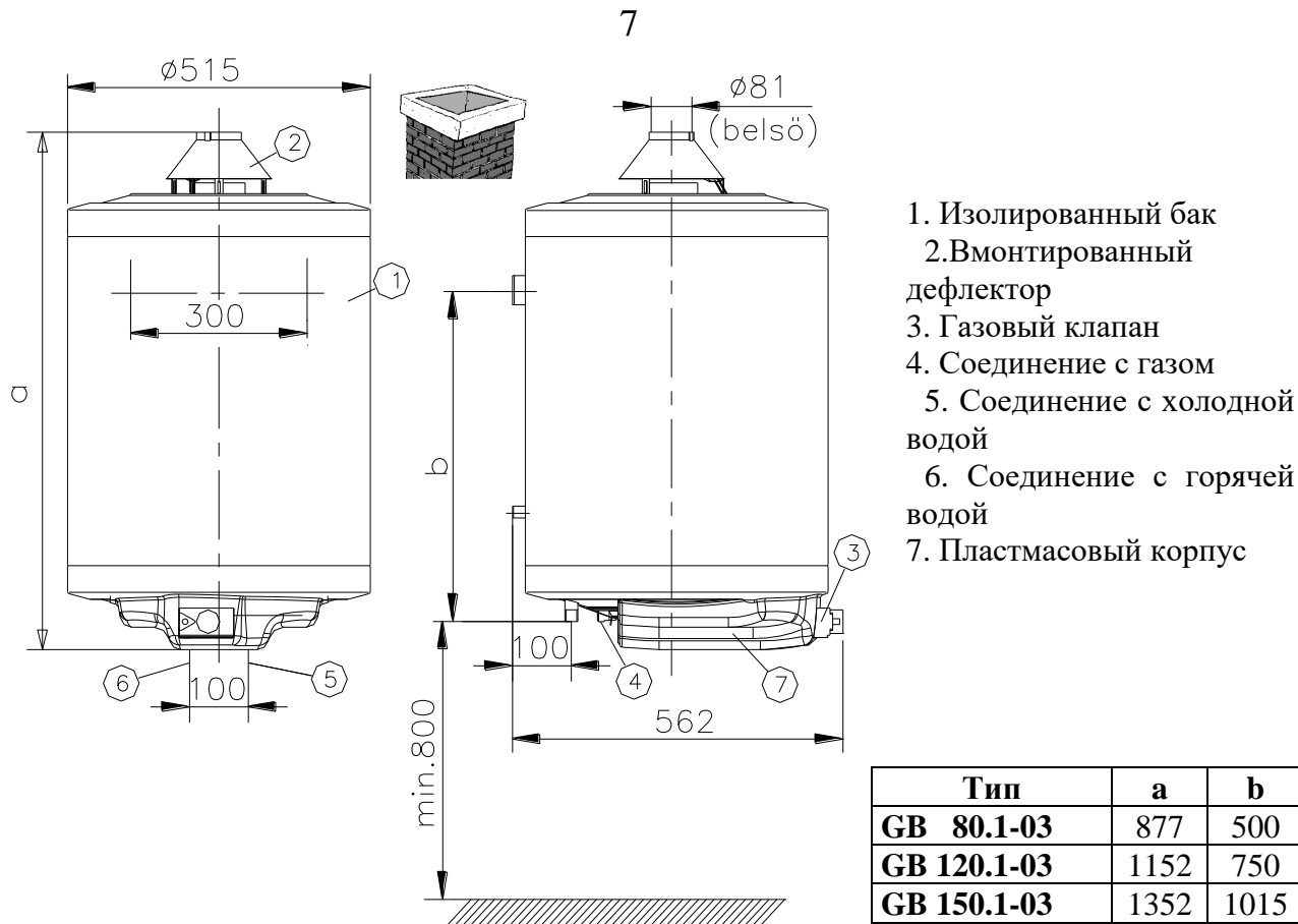
Схема № 1.1 - Общий вид с габаритными размерами
