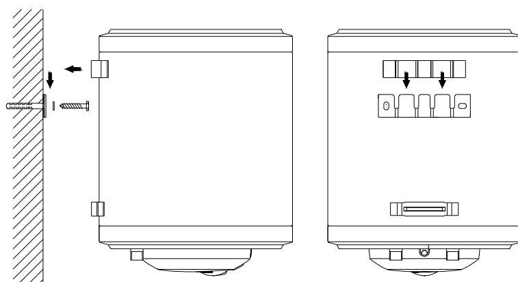
2. schéma
