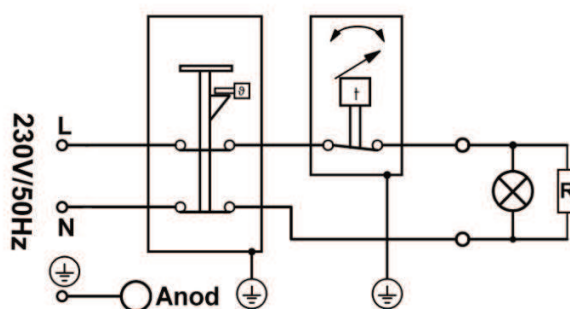
Schéma zapojení
