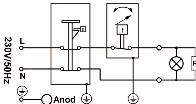
Kapcsolási vázlat
