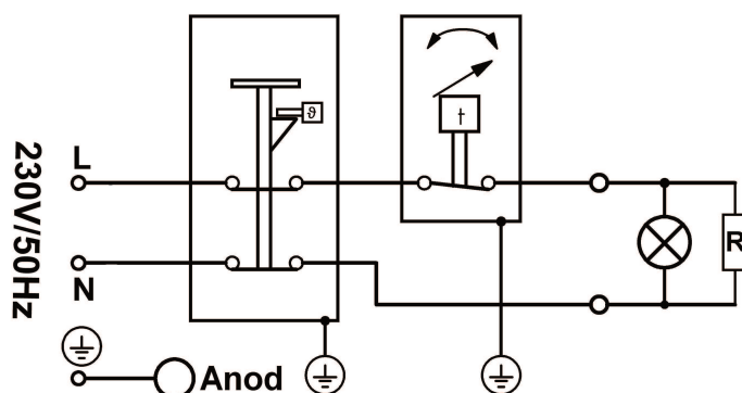
Схема подключений
