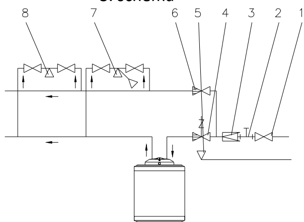
4. schéma
