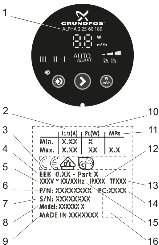
18. ábra Adattábla
