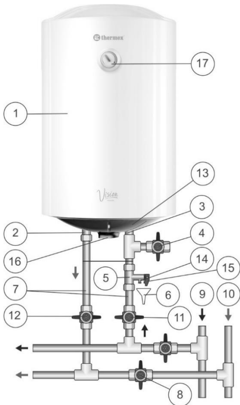
1. ábra. Az elektromos vízmelegítő csatlakoztatási ábrája a vízellátáshoz
