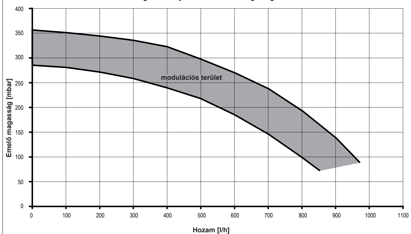
Keringetőszivattyú maradék emelő magassága 4 m
