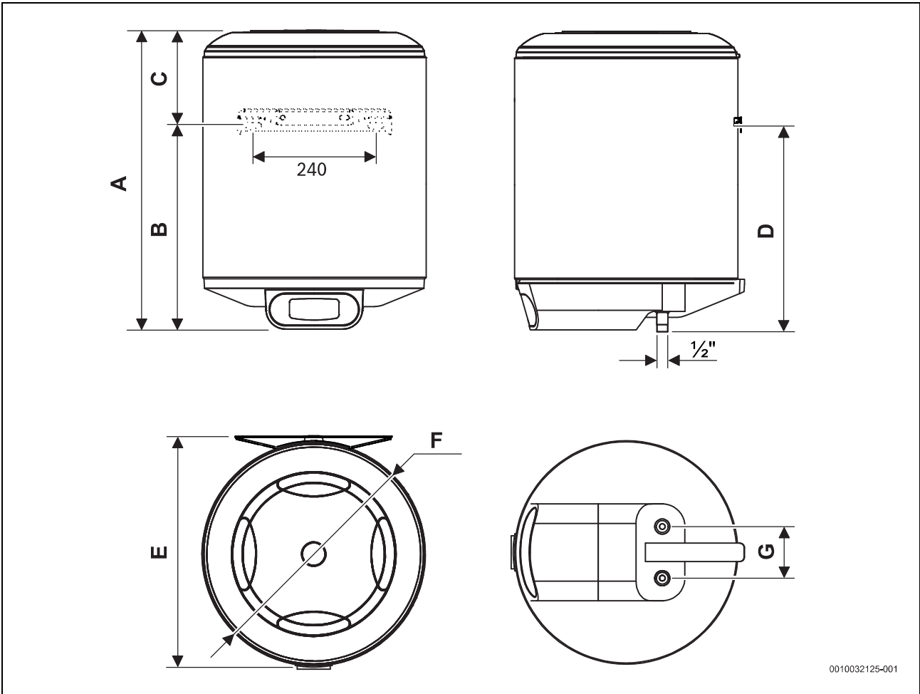
2. ábra Méretek mm-ben (fali akasztós, függőleges szerelés)
