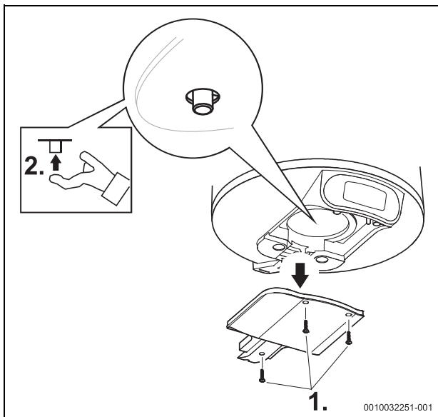
12. ábra Biztonsági hőmérséklet-határoló
