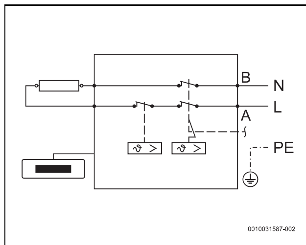
13. ábra Csatlakoztatási rajz
