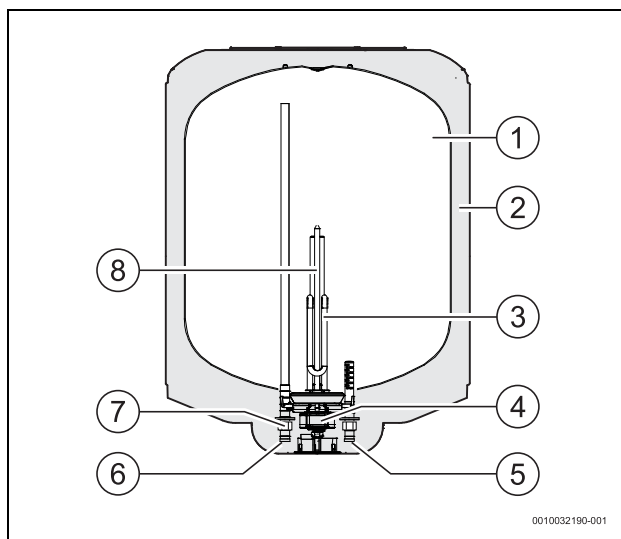
3. ábra A készülék komponensei
