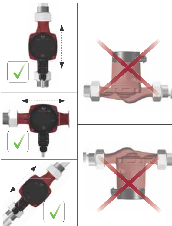
1. ábra A GRUNDFOS ALPHA1 L beépítése
